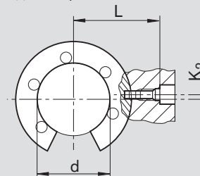
Вал диаметром 30, 40, 50
