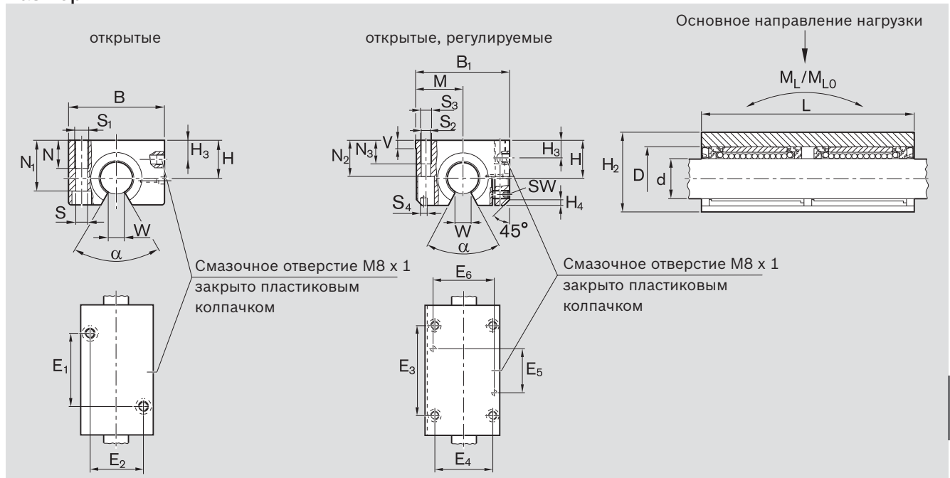
Размеры (мм)
