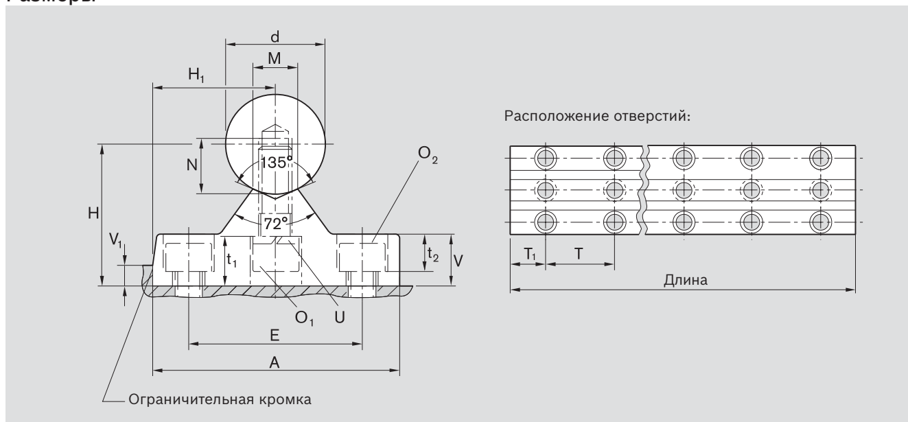
Размеры (мм)
