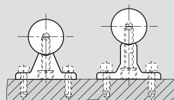
традиционные направляющие с фланцем
