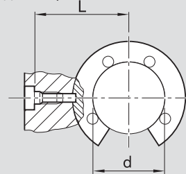
Вал диаметром 16
