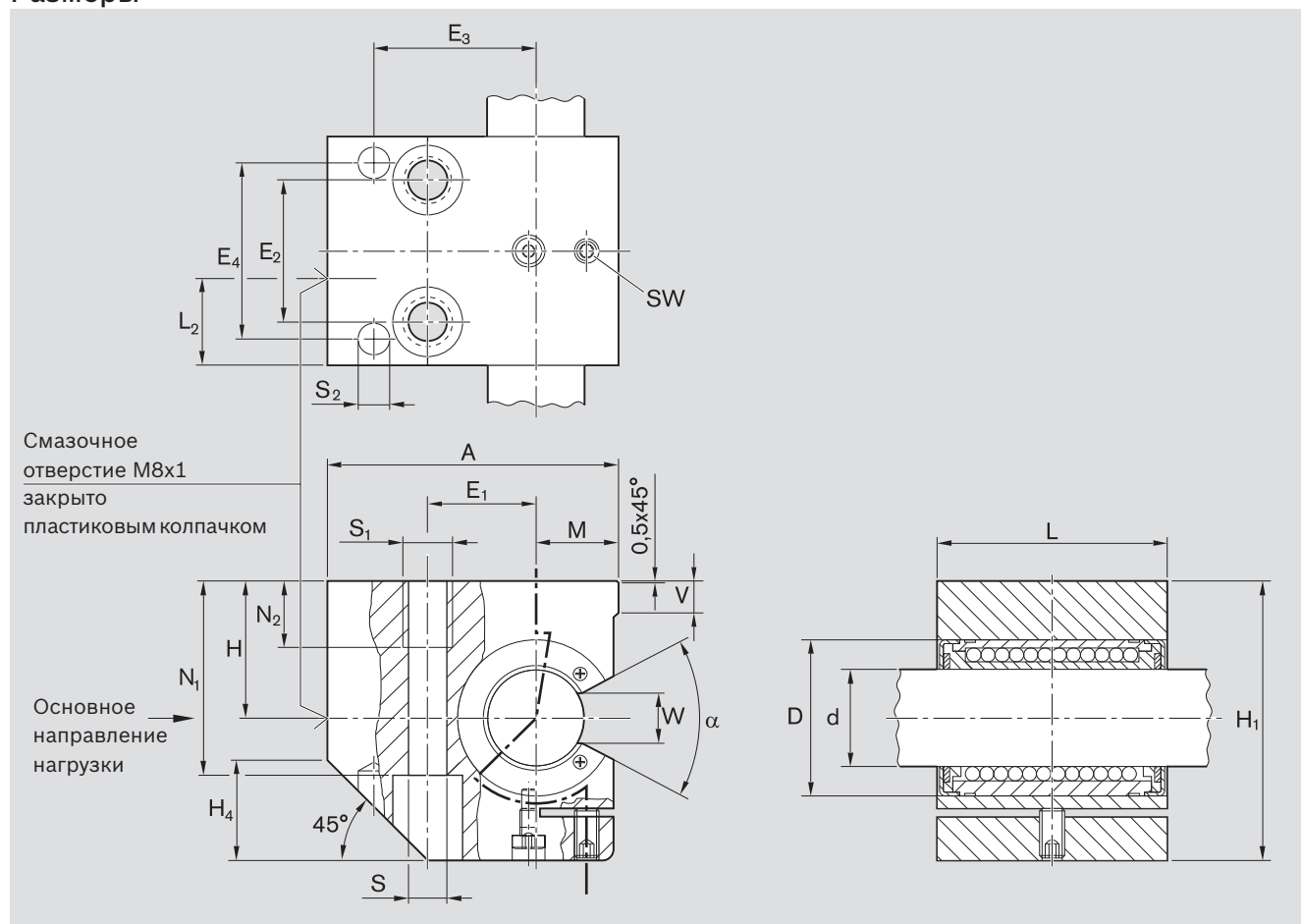
Размеры (мм)
