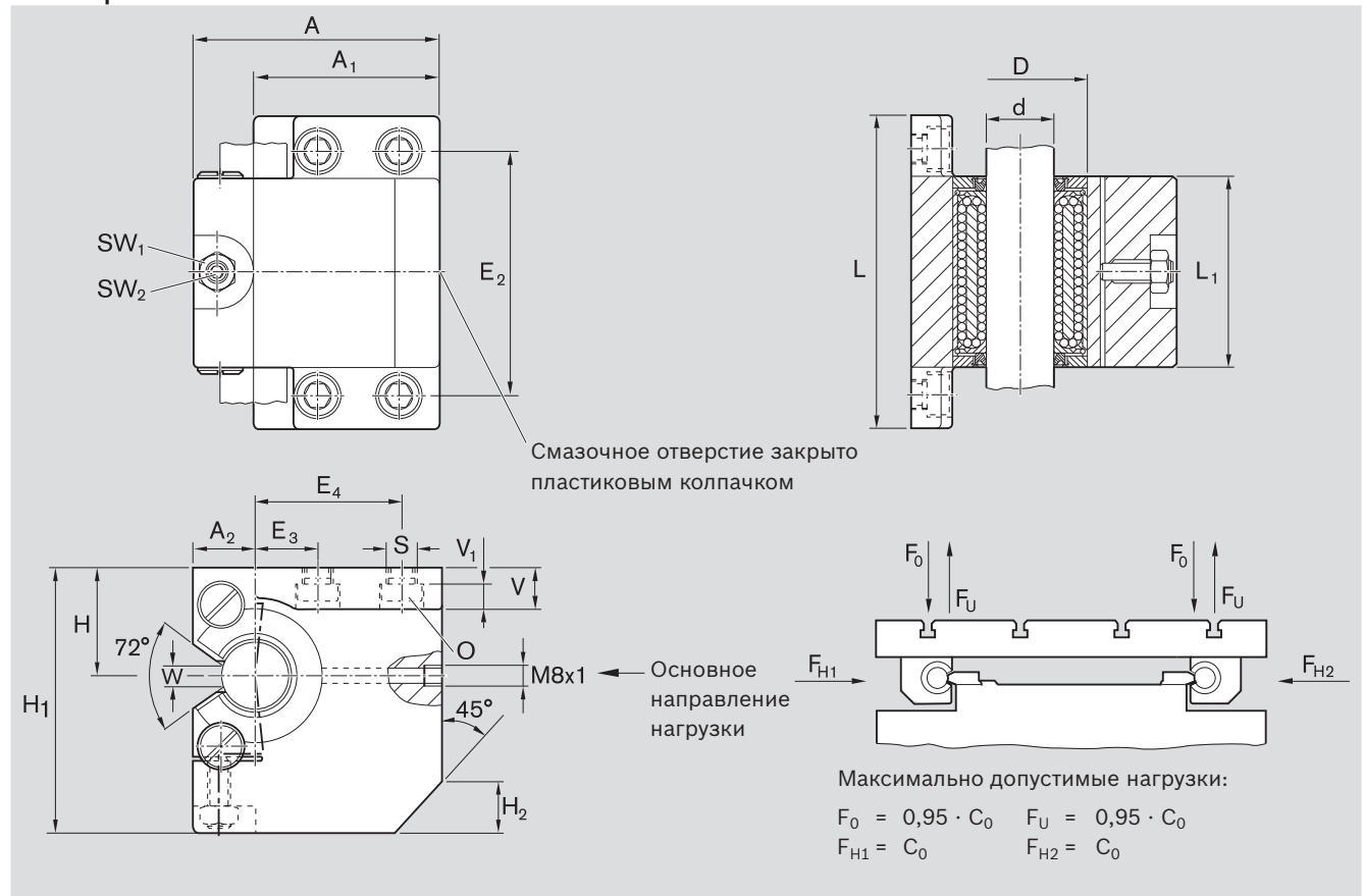
Размеры (мм)
