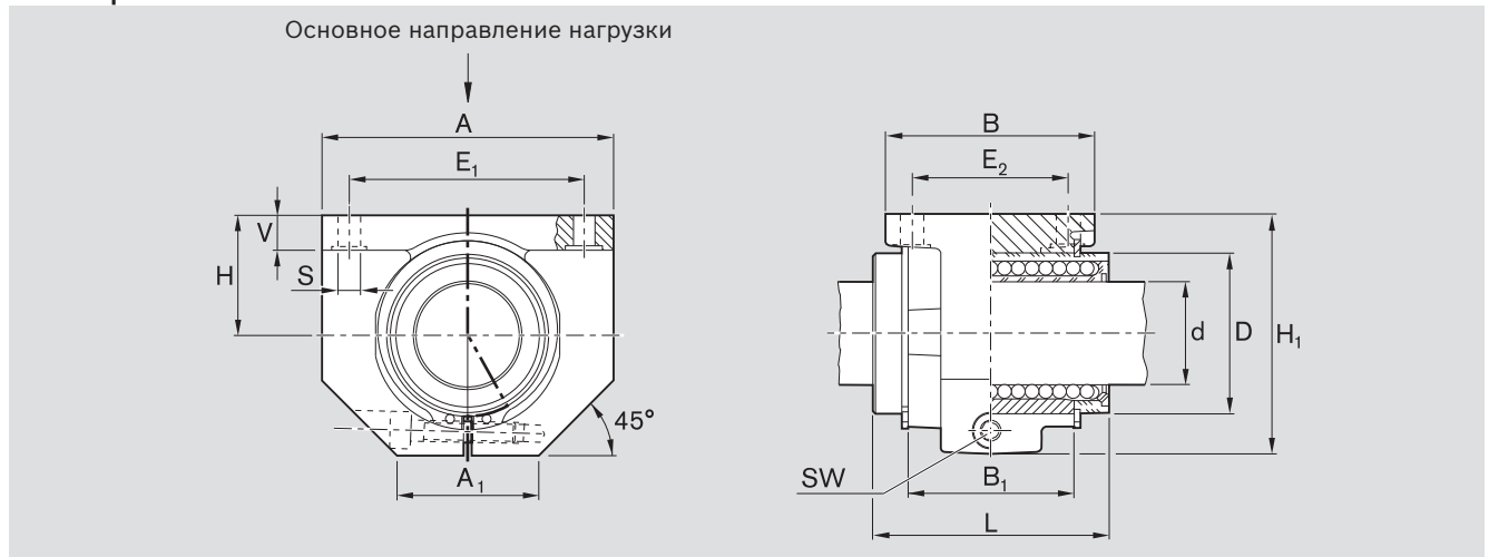
Размеры (мм)
