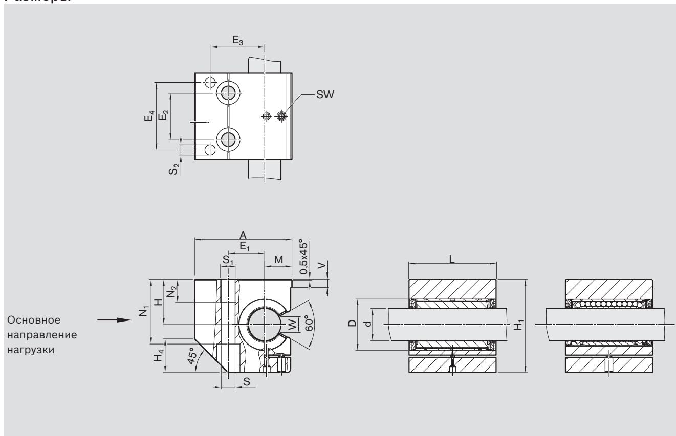
Размеры (мм)
