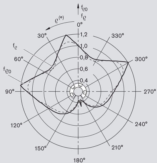
Вала диаметром 12
