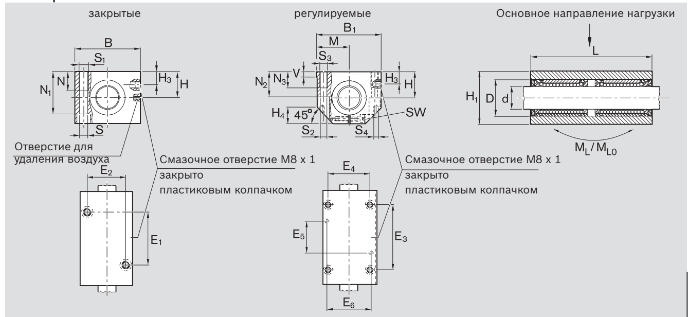
Размеры (мм)
