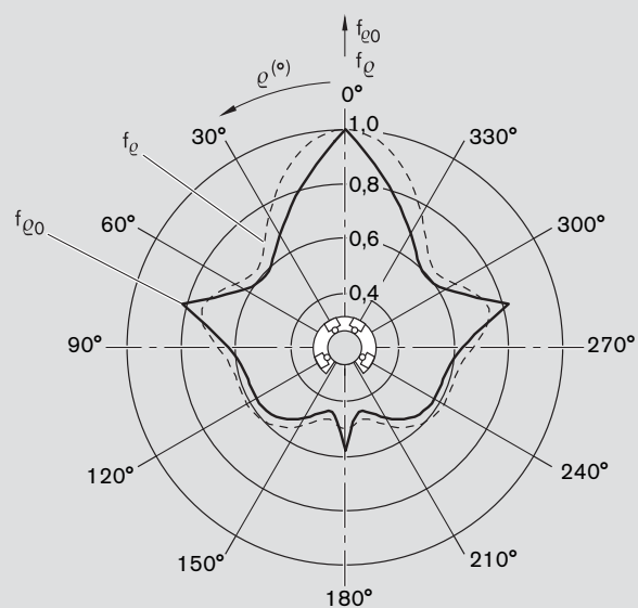
Вал диаметром 16
