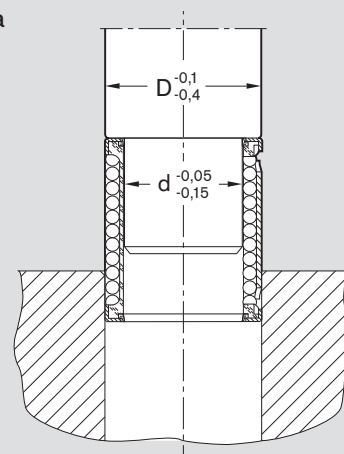
Монтажная оправка
