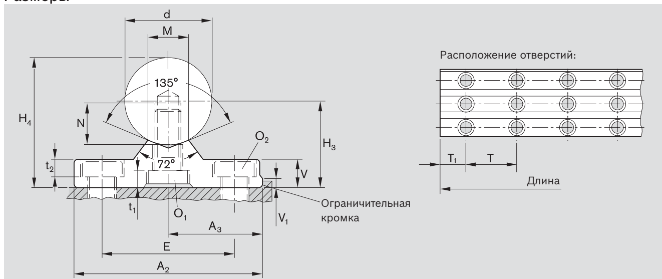
Размеры (мм)
